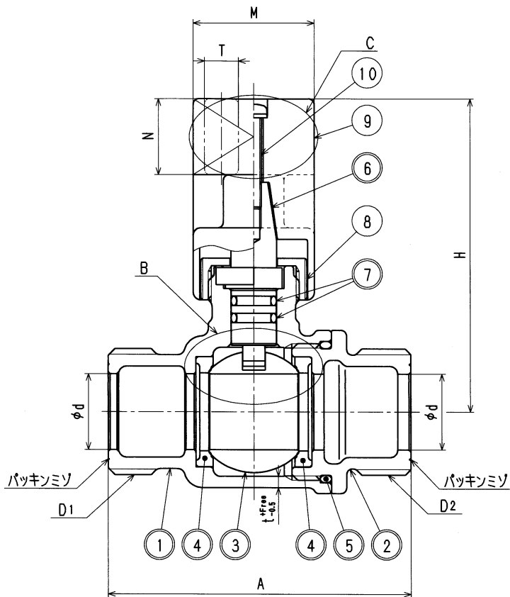
寸法表
